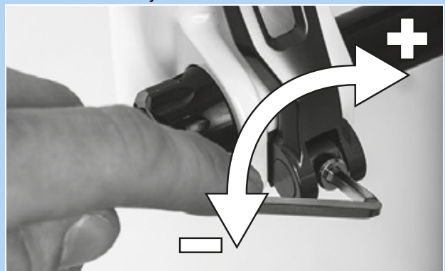
194. ábra: A gyorszár szorítóerejének beállítása
