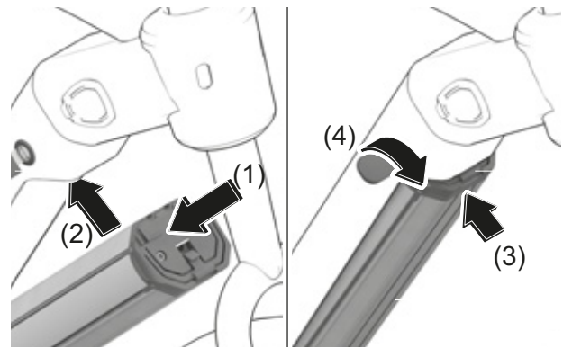
144. ábra: Akkumulátor beszerelése
