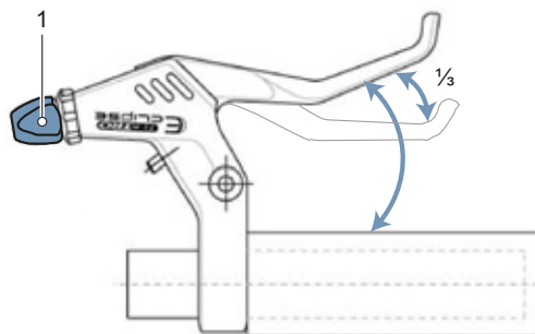
165. ábra: Fordítsa el az állítócsavart (1), amíg a fékek a kézifék 1/3-nyi mozgása után be nem kapcsolódnak
