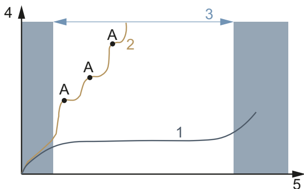
158. ábra: Kopás, üzemidő (x) az anyagledörzsölődés (y) arányában diagram
