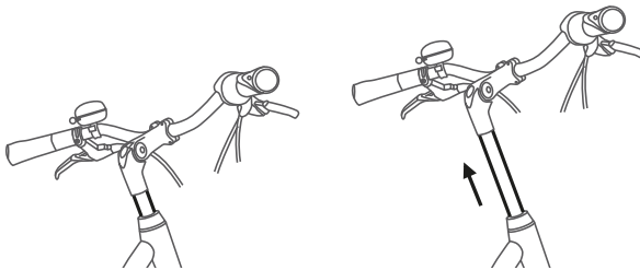
111. ábra: Szárcsöves kormányszár magasságának állítása
