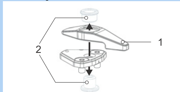
82. ábra: Rögzítőkar összekötése az alaplemezrel
