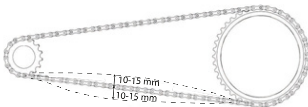
166. ábra: Példa láncfeszítés ellenőrzésére: 5 mm felfelé, 10 mm lefelé = 15 mm eltérés
