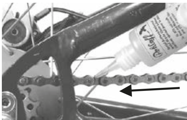
159. ábra: Lánc kenése
