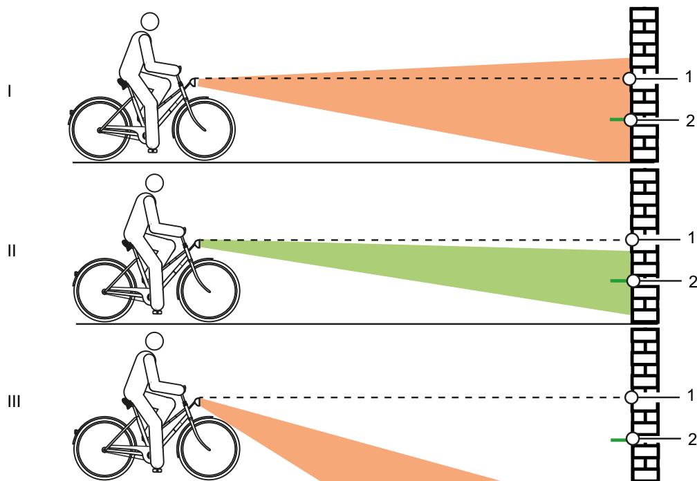
129. ábra: Túl magasra (1), helyesen (2) és túl mélyre (3) beállított világítás
