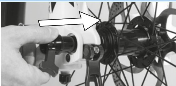
69. ábra: A kereszttenyely betolása nyílrányban
