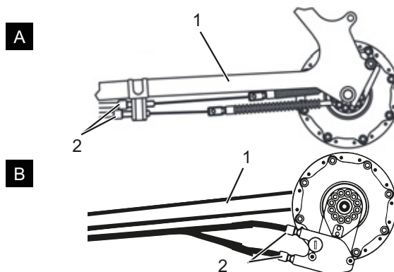
191. ábra: Beállítóhüvelyek (2) láncvillára (1) szerelt bovdenes működésű, kétbovdenes váltó két alternatív kivitelén (A és B)
