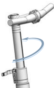
138. ábra: Példa: All Up egyenesbe állítva
