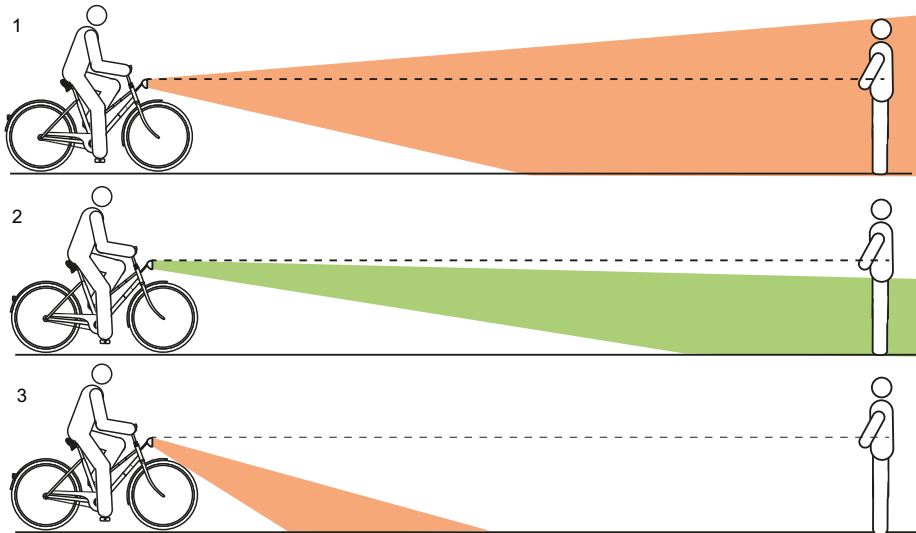
127. ábra: Túl magasra (1), helyesen (2) és túl mélyre (3) beállított világítás
