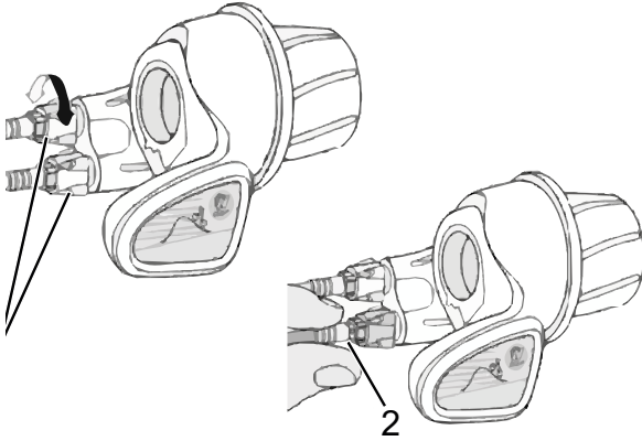
192. ábra: Forgómarkolatos váltó beállítóhüvelyekkel (1) és a váltó (2) játéka
