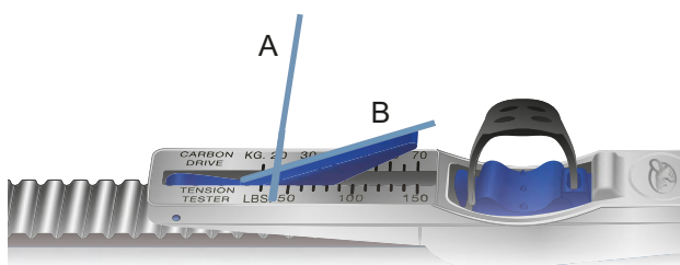
183. ábra: Leolvasott érték példája: 20 kg
