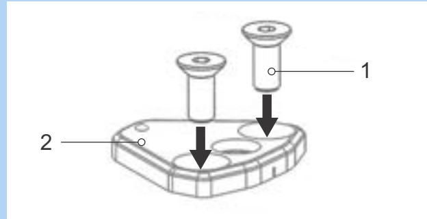
81. ábra: Süllyesztett fejű csavarok bedugása az alaplemezbe
