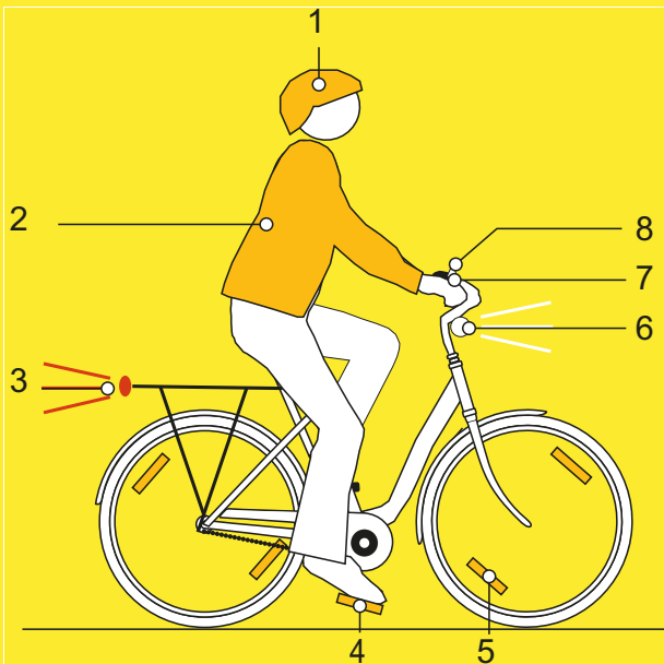
135. ábra: Közlekedésbiztonság
