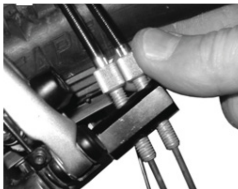
189. ábra: Belső váltóvezérléssel rendelkező ROHLOFF agyváltozatok húzásbeállítója a húzásellentartón van
