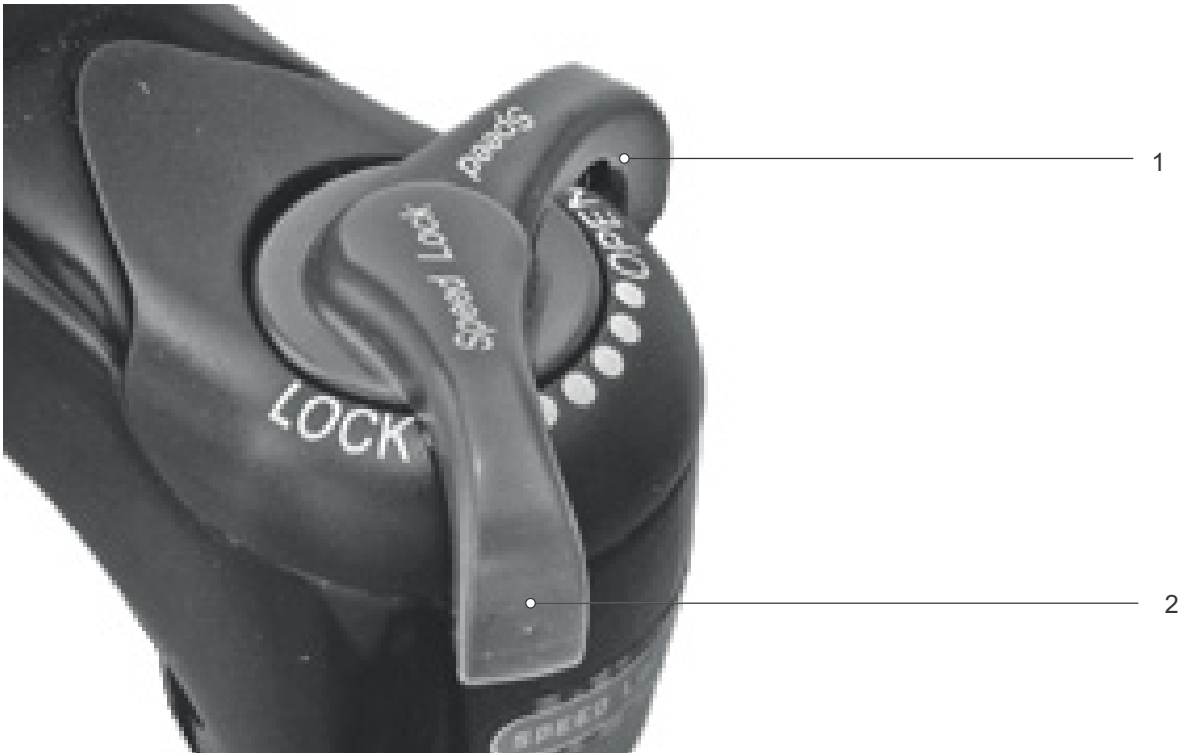
151. ábra: SR SUNTOUR nyomásfokozat-lengéscsillapító nyitott (1) és zárt (2) helyzetben
