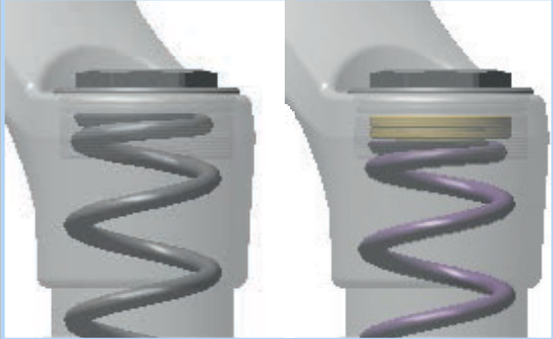
Abbildung 113: Vorspannungseinstellung hinein und heraus drehen.
