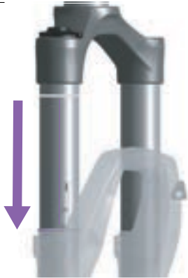
Abbildung 110: O-Ring an der Federgabel verschieben
