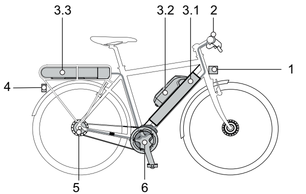
Abbildung 38: Schema elektrisches Antriebssystem mit elektrischen Bauteilen
