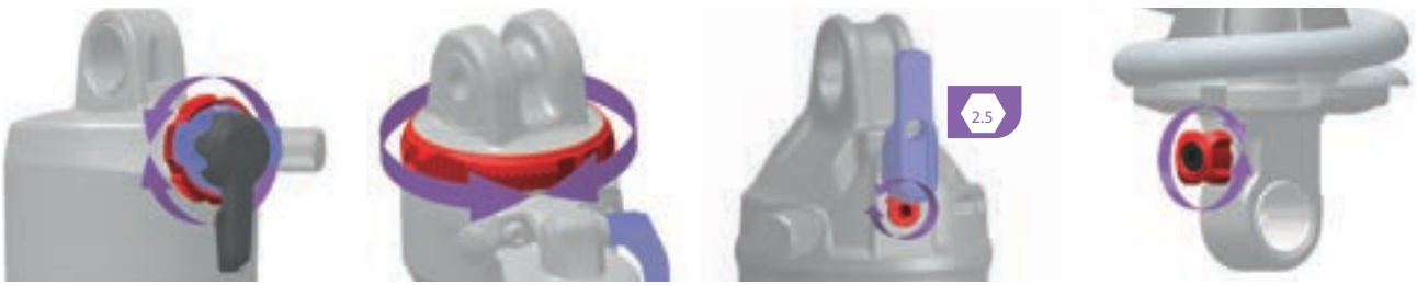
Abbildung 120: Lage und Form des Zugstufeneinstellers (rot) ist abhängig vom Modell
