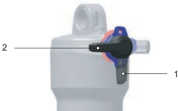
Abbildung 124: Offenen Position (1) und Schwellenposition (2) des Hebels
