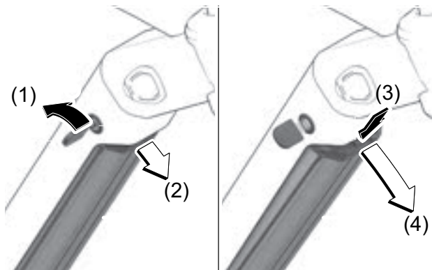
Abbildung 136: Integrierten Akku herausnehmen
