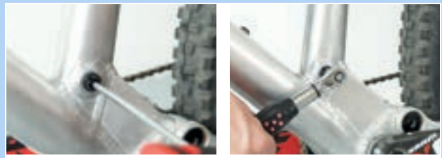
Abbildung 231: Sattelstütze festschrauben
