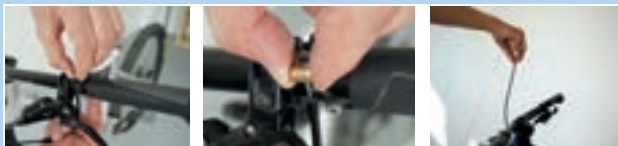
Abbildung 209: Fernbedienung lösen
