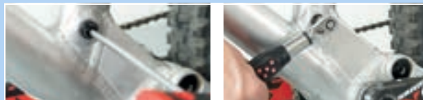
Abbildung 200: Postpin Achse befestigen
