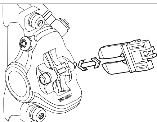
Abbildung 48: Transportsicherung befestigen
