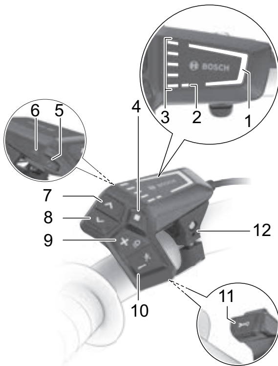
Abbildung 139: Übersicht Bedieneinheit BOSCH LCD Remote
