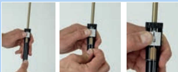
Abbildung 175: Seilzug aushängen
