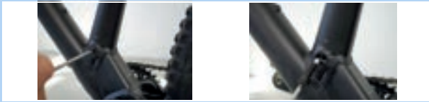
Abbildung 208: Sattelstütze lösen
